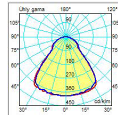
uhol svietenia 90°
