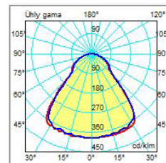
uhol svietenia 90°
