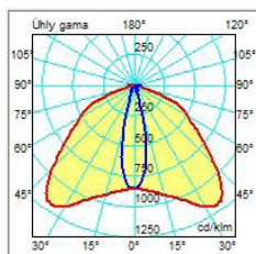
Abstrahlwinkel 26 x 108°
