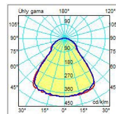
Abstrahlwinkel 90°
