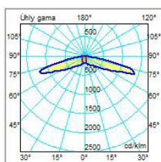
Abstrahlwinkel 80° x 155°
