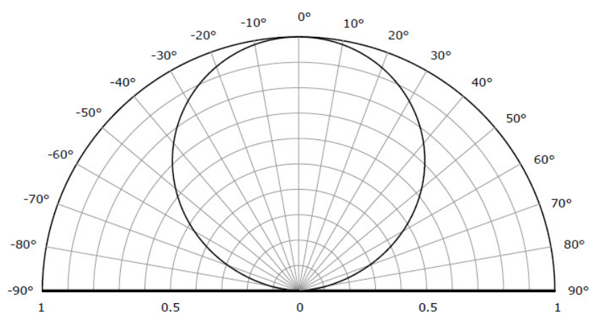
uhol svietenia 120°
