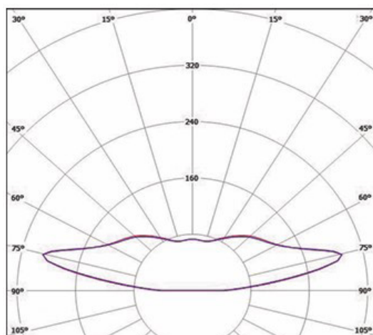
uhol svietenia
